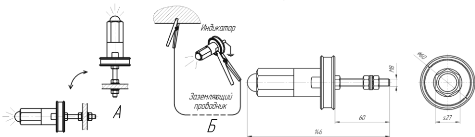
Рисунок 3 - Установка устройства
